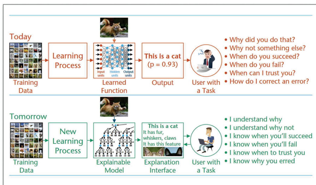
Figura 1 – Conceito de XAI
